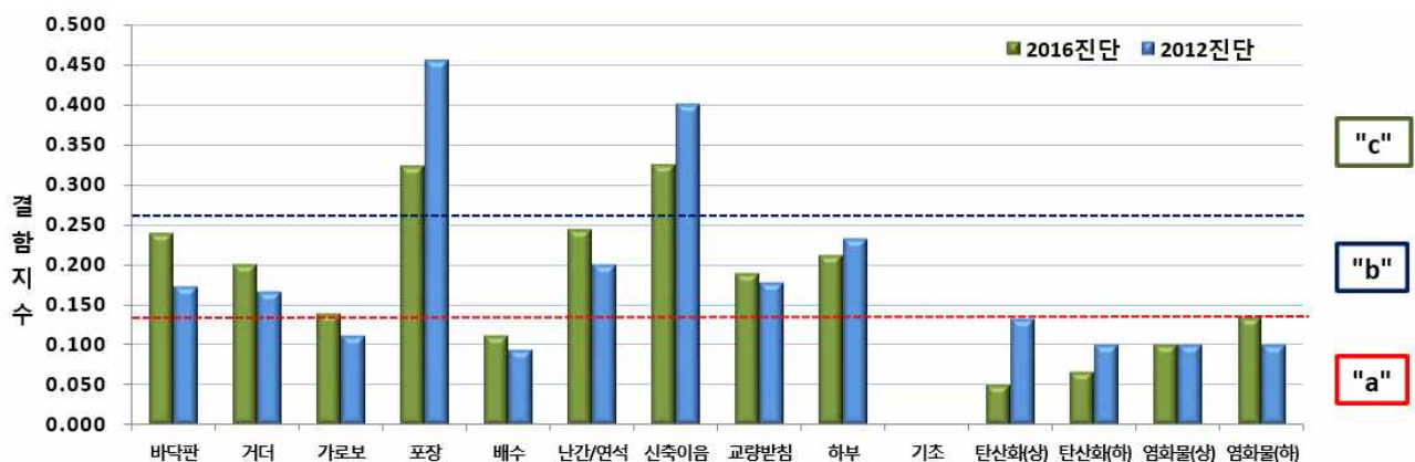
【그림 4.2】 기 진단 결과와의 부재별 상태평가 결과 비교
